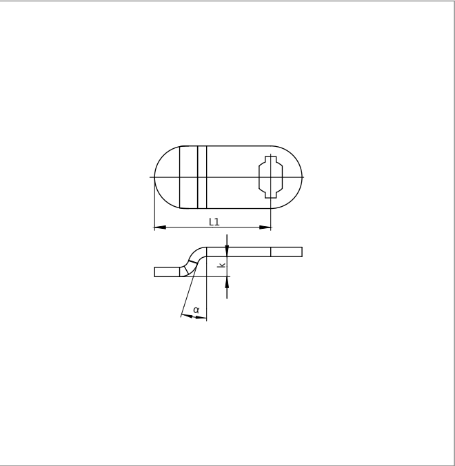
Schließhebel gebogen
