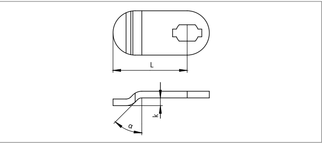
Schließhebel gebogen
