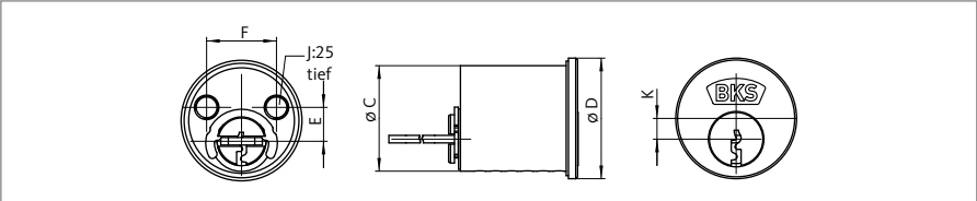
Befestigungsgewinde bei Außenzylindern
